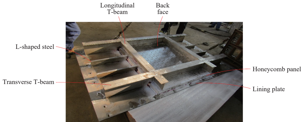
图 2 实验样件
