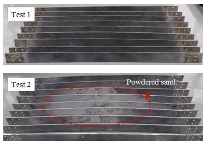
图 16 靶板变形形貌对比
