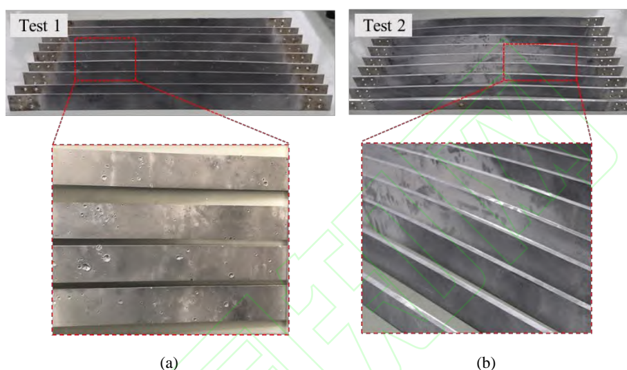
图 18 砂土对靶板的侵彻作用：(a) 试验 1 (b) 试验 2
