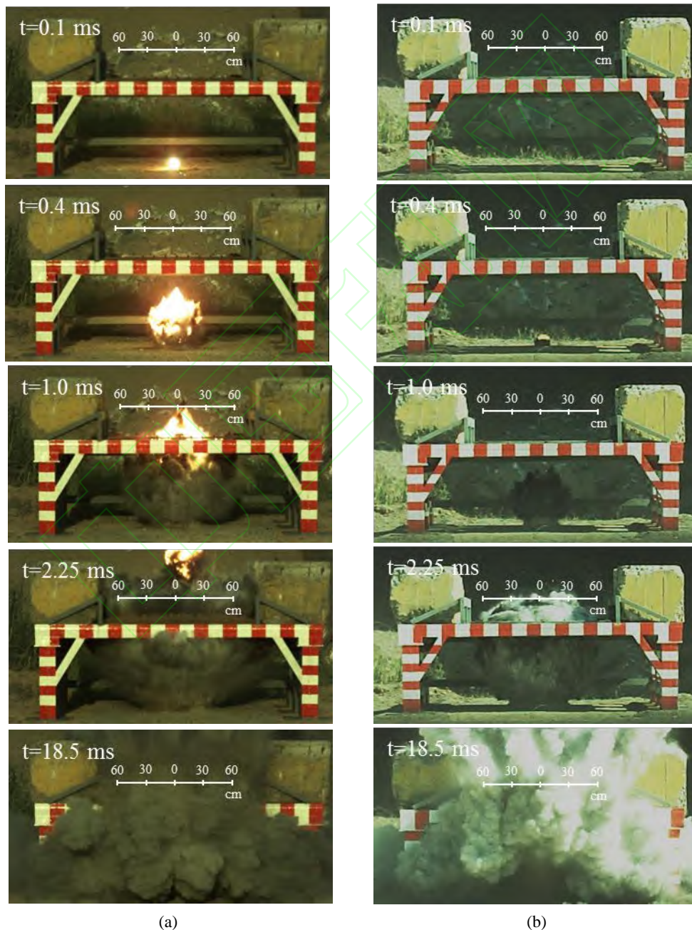
图 9 爆炸过程：(a) 试验 1，(b) 试验 2
