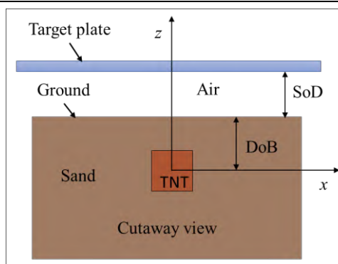
图 7 炸药、砂土、靶板的相对位置 Fig. 7 Relative position of explosive, sand and target plate
