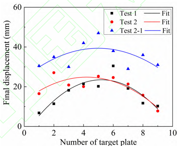
图 14 靶板的变形挠度
