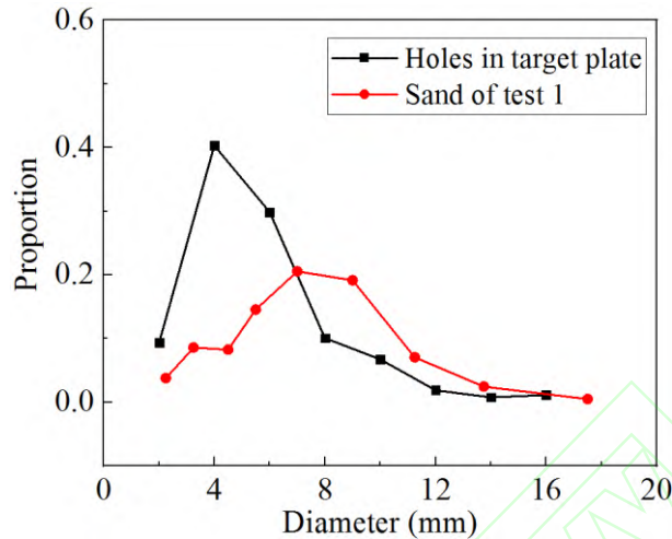
图 20 不同直径凹坑与砂子所占比例
