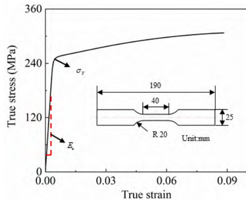
图 3 AL6063 真实应力-应变曲线
