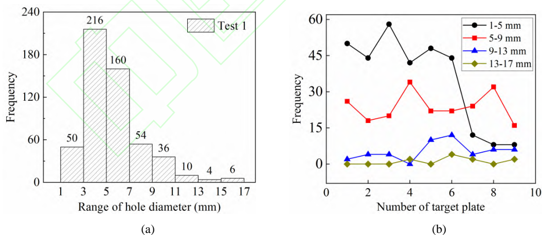
图 19 试验 1 靶板上凹坑数量统计：(a) 不同直径凹坑频数分布 (b) 靶板上凹坑频数分布
