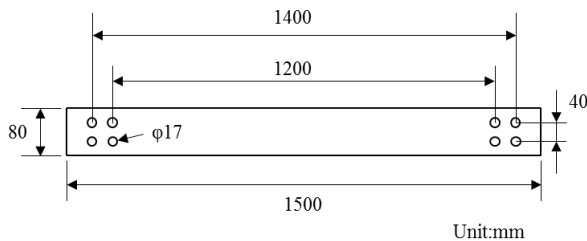
图 2 靶板平面尺寸
