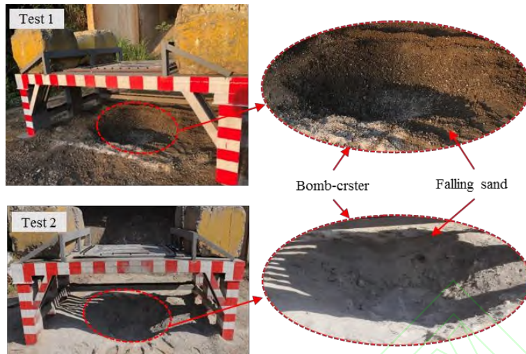
图 15 试验 1 和试验 2 产生的炸坑形貌
