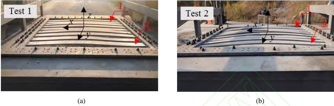
图 12 靶板变形 (a) 试验 1 (b) 试验 2
