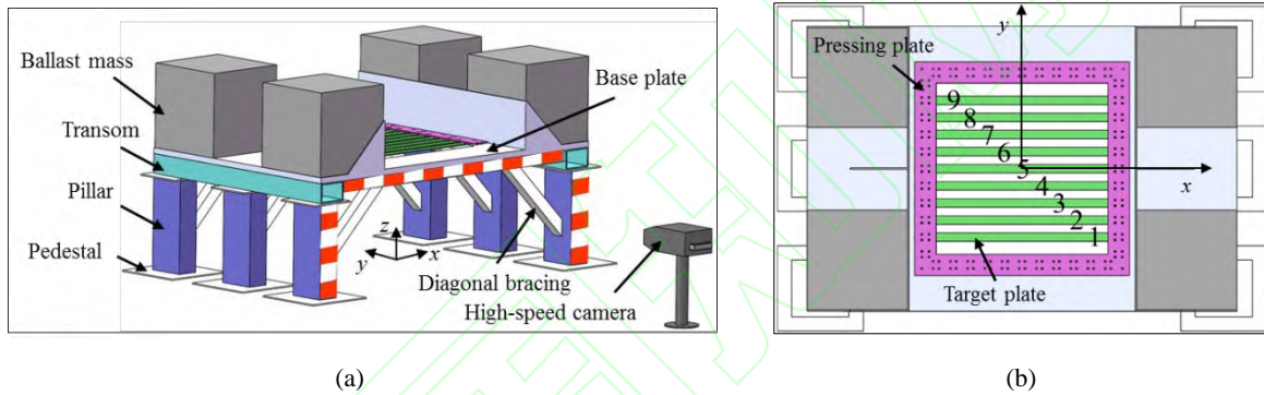
图 1 试验工装: (a) 斜视图 (b) 俯视图
