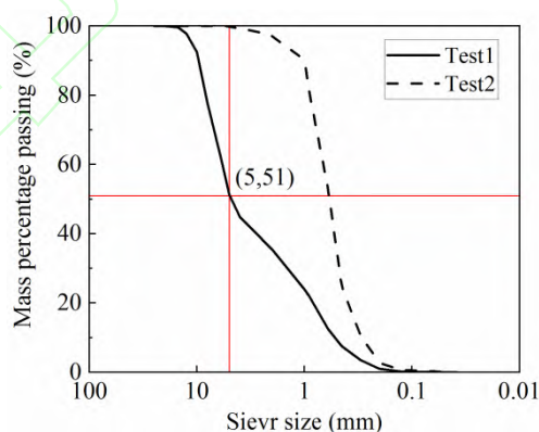
图 5 试验 1 和试验 2 采用砂土的粒径分布
