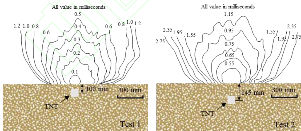
图 17 试验 1 和试验 2 中爆炸产物和砂土的喷射轨迹对比
