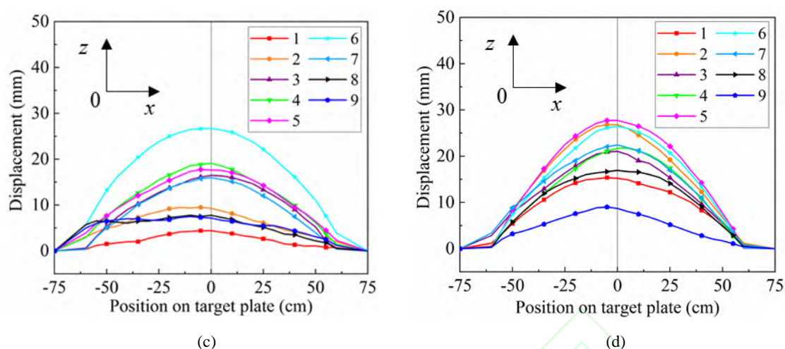
图 13 靶板变形轮廓 (a) 试验 1 (b) 试验 2 (c) 试验 1 (d) 试验 2
