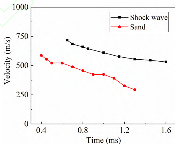
图 11 冲击波与砂土的速度时程曲线
