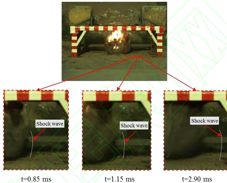
图 10 冲击波横向传播过程(为清晰标识冲击波位置，图中用虚线标注波阵面位置)
